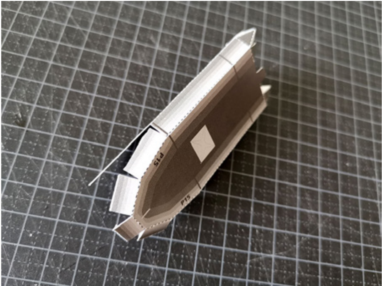
44) Snij onderdeel 29 uit en vouw langs de vouwlijnen.
